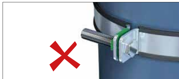
Неправильно затянутый хомут
