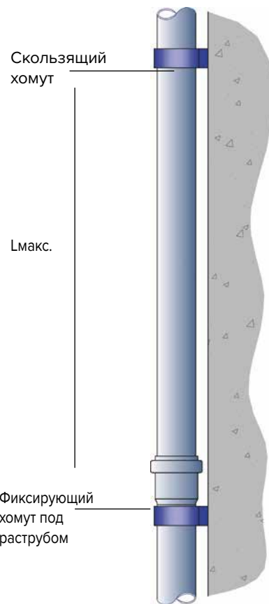
Вертикальная прокладка труб
