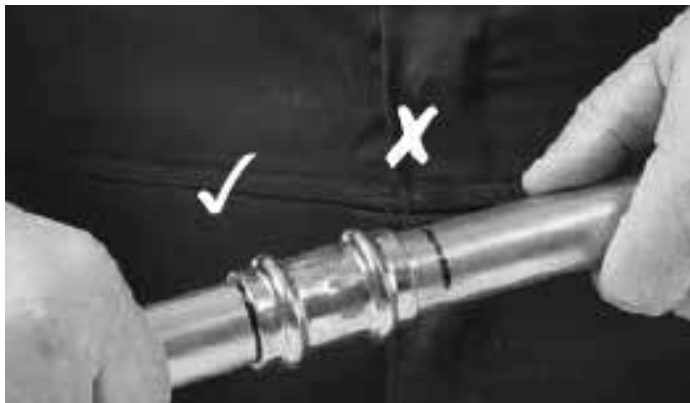
Сборка трубы с фитингом.
