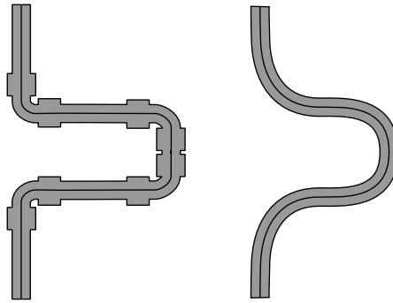
П-образный изгиб трубы или трубопроводный компенсатор.
